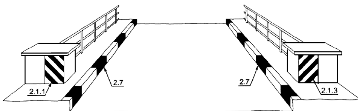
Рисунок В.21 - Пример нанесения разметки 2.1.1, 2.1.3 и 2.7
