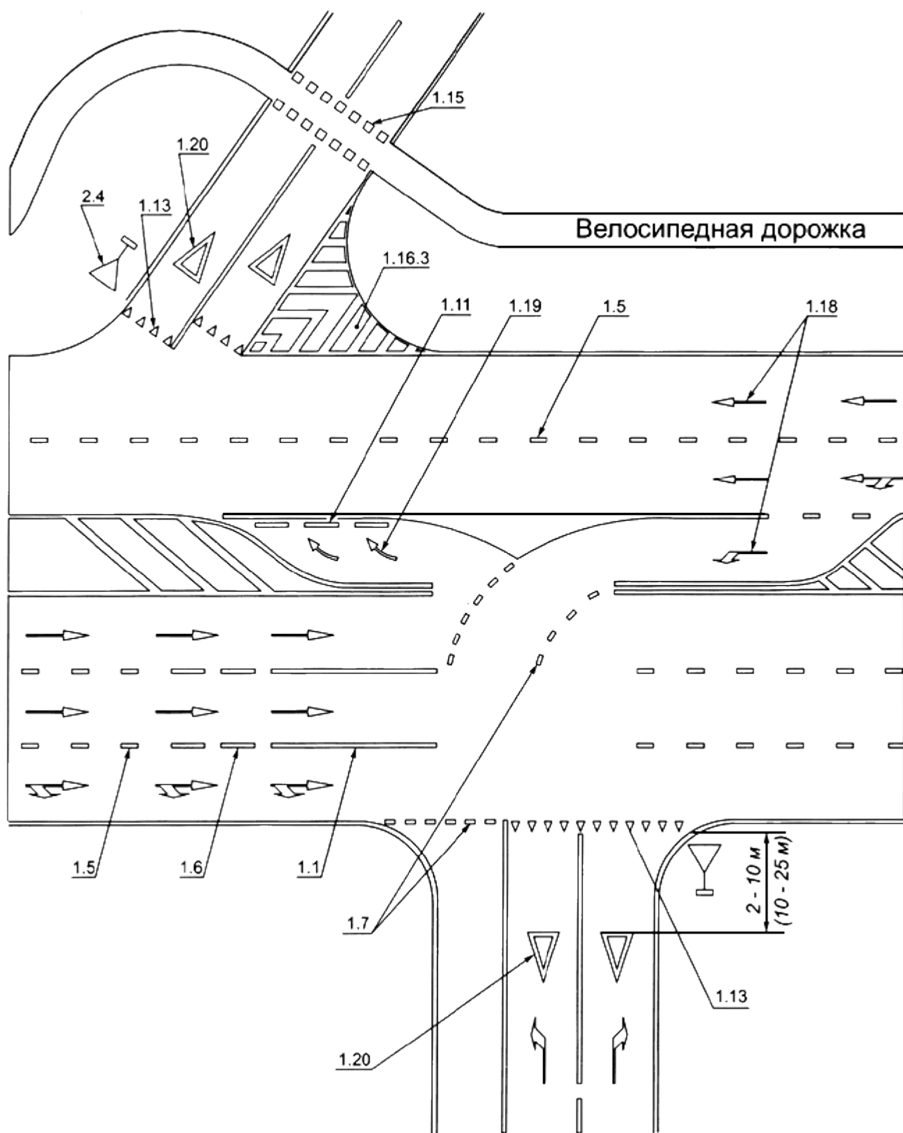
Рисунок В.10 - Пример нанесения разметки канализированного пересечения
