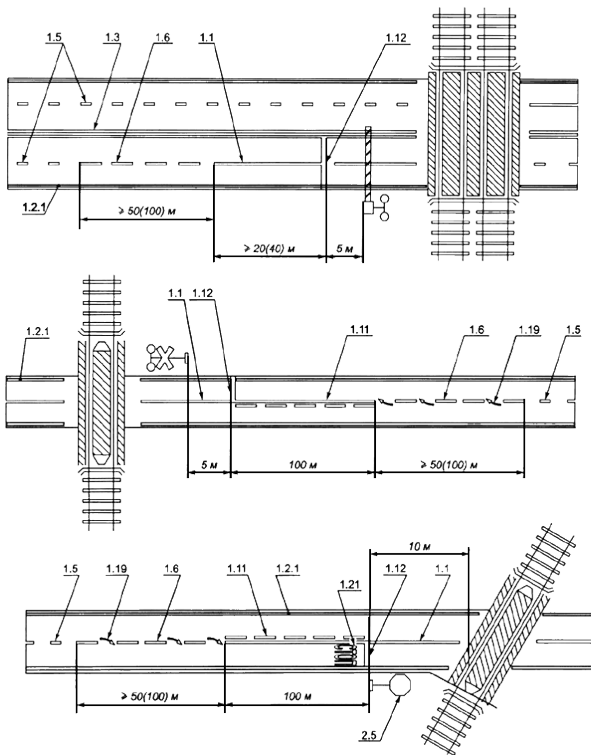
Рисунок В.17 - Пример разметки участка дороги на подъезде к железнодорожному переезду
